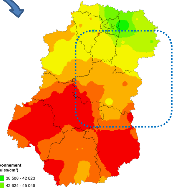
Cumul du rayonnement du 25/05/2016 au 25/06/2016
